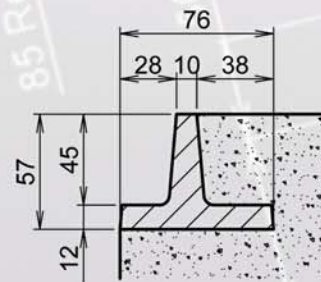
Section A-A Typ Frame
